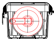
b) Sezione \phi max 190
