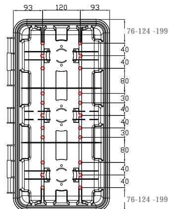
c) 22 punti di fissaggio rinforzati
